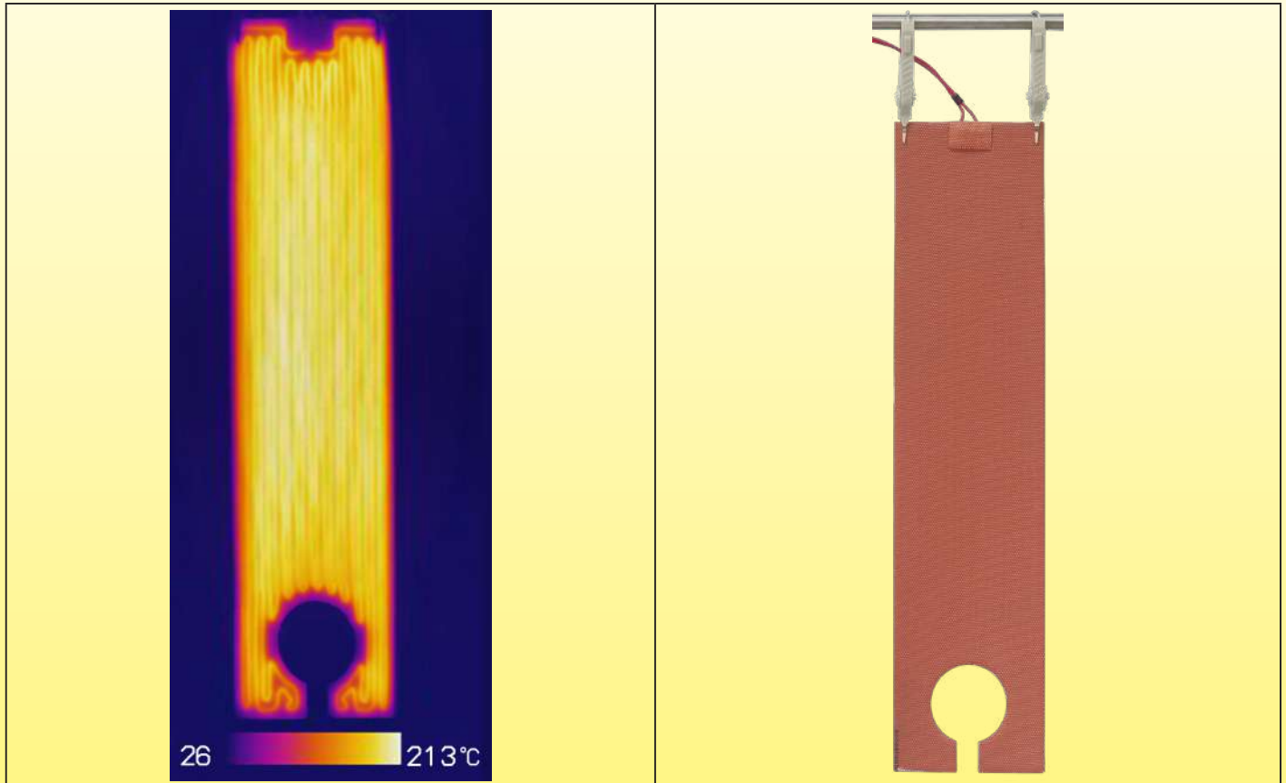
Image thermographique d'une résistance chauffante plate silicone épaisseur 2,4mm chargée à 1W/cm^2 , suspendue dans l'air calme, non fixée sur une paroi, à une température ambiante de 25^{\circ}C . La température de surface atteint 213^{\circ}C , soit une valeur proche de la destruction.
